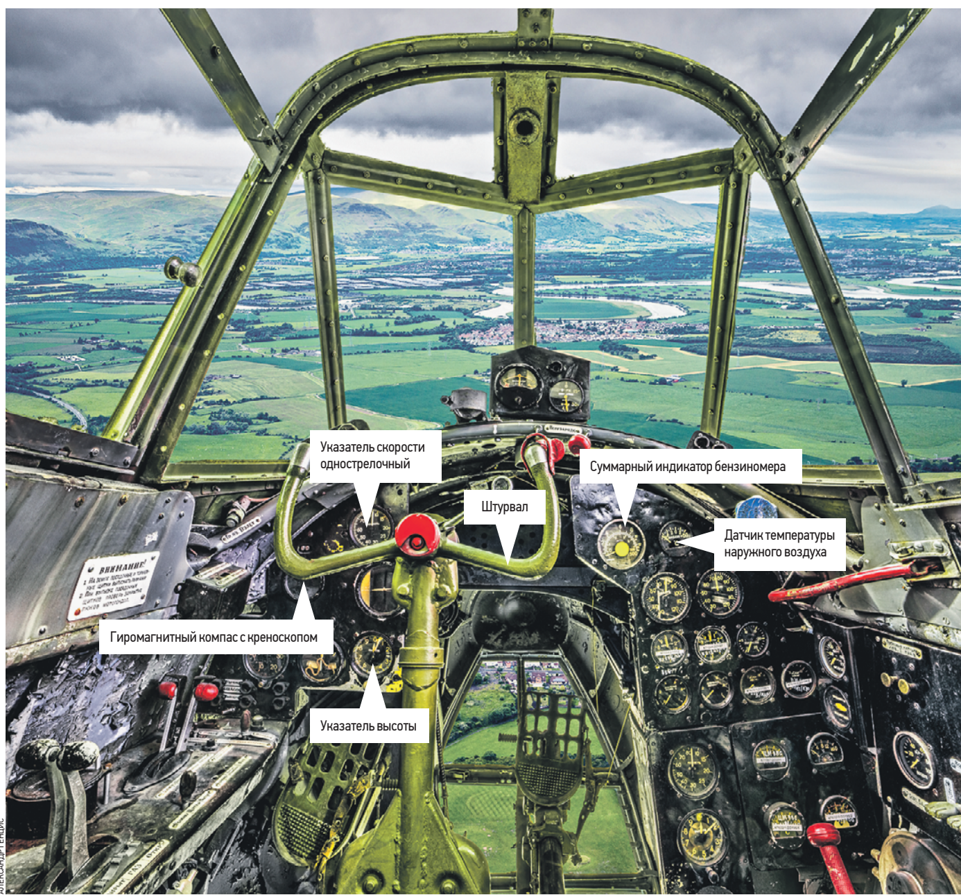
Вчера 12:20 Снимок кабины пикирующего бомбардировщика Пе-2 времен Великой Отечественной с выставки, организованной Александром Генцисом. Благодаря высокой детализации можно разглядеть все приборы и их показания
